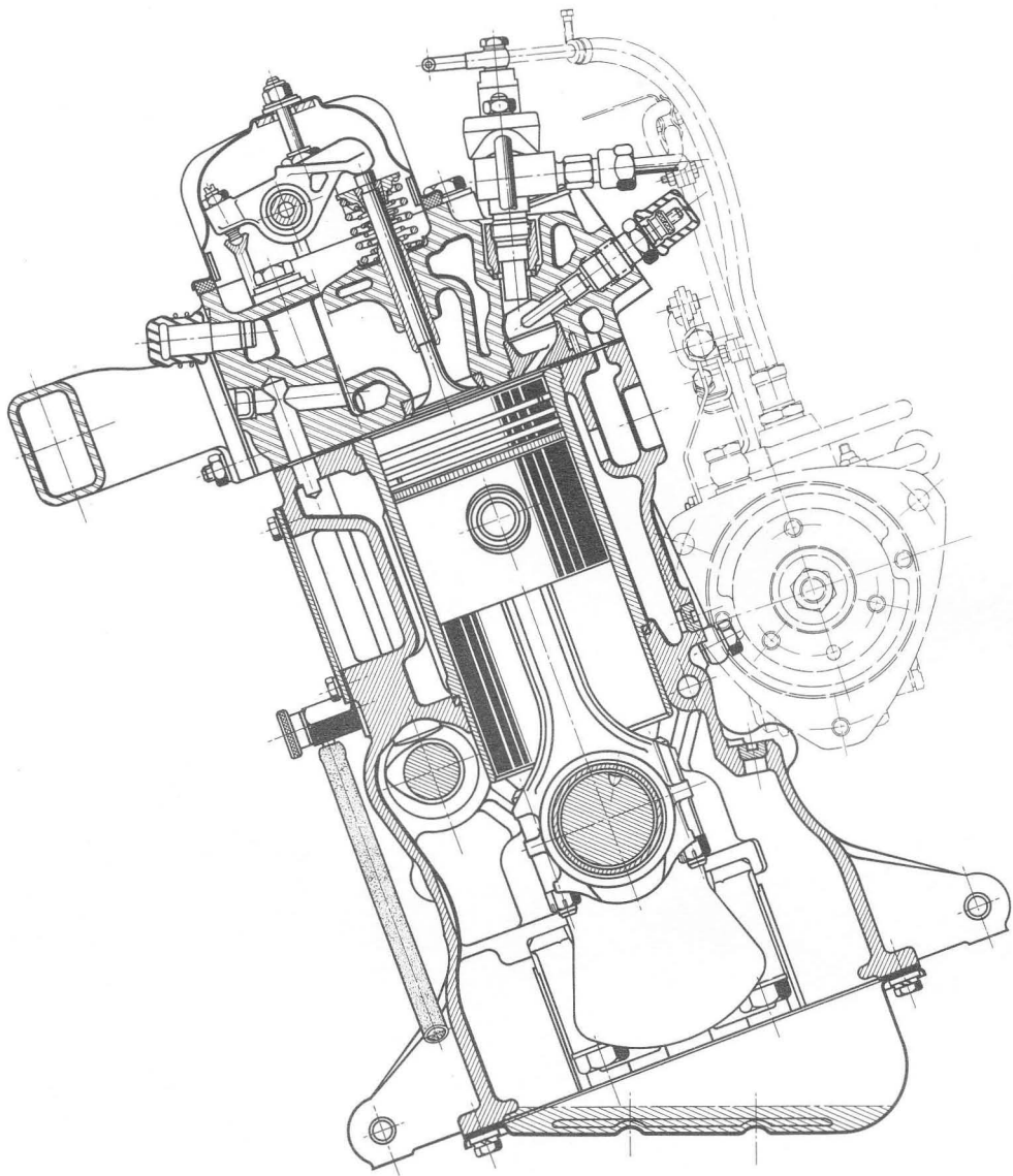
COUPE TRANSVERSALE
